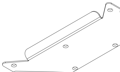
U021 Qty 1
